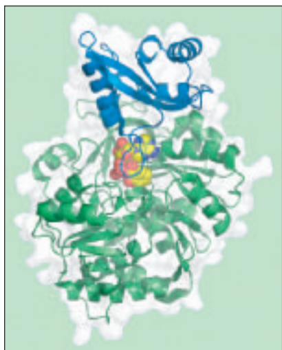
Die Abbildung zeigt die dreidimensionale Struktur des Proteins DhhE, das für bestimmte Bakterien lebensnotwendig ist. Aus der Struktur lässt sich seine Funktionsweise ableiten, die die Basis für die Entwicklung neuer Antibiotika liefern kann. Abbildung: MLU
